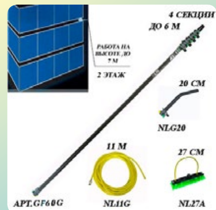
Комплект для мытья окон на высоте до 7 м (2 этаж) nLite Starter Plus
