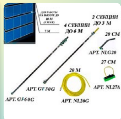
Комплект для мытья стекол на высоте до 10 м (3 этаж) nLite Beginner Plus
