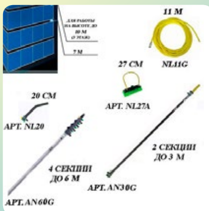
Комплект для мытья окон на высоте до 10 м (3 этаж) nLite Beginner Econom
