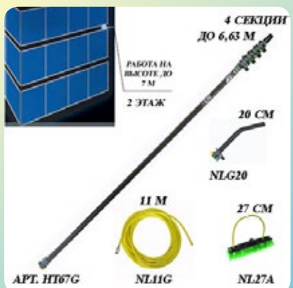
Комплект для мытья окон на высоте до 7 м (2 этаж) nLite Starter Optimal
