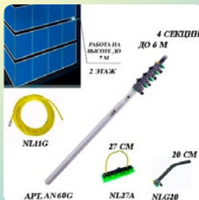
Комплект для мытья окон на высоте до 7 м (2 этаж) nLite Starter Econom
